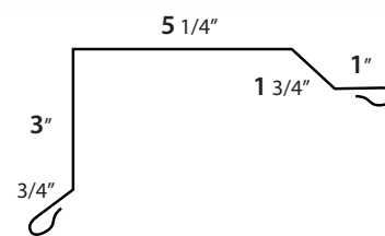
RAKE
